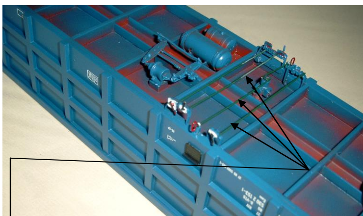
K: remschakelstangen (3x) / Bremsschaltergestang (3x)
